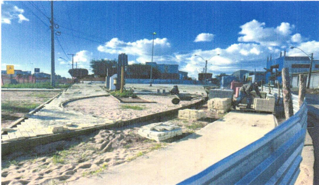
FOTO 05 – Pavimentação em bloco de concreto vibroprensado, intertravado, colorido, 10x20cm, e=6cm, 46un/m 2 , NBR9781, Fck(min)=35MPa, sob coxim areia grossa compactada c/ placa vibratória, e(comp.)=6cm, rejuntado c/ areia fina
